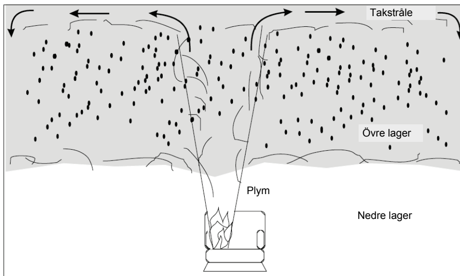
Figur 4 Zonmodellens uppbyggnad.
